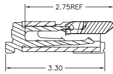
Section A-A Scale 2:1
