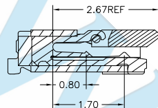
Section B-B Scale 2:1
