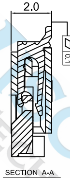
SECTION A-A
