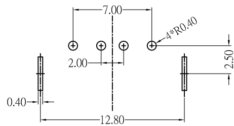
LAYOUT P.C.B
