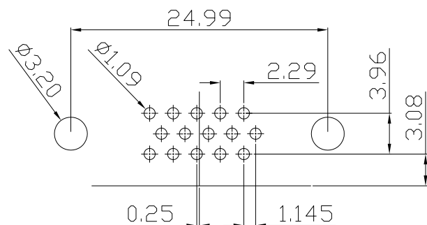
P.C.B. LAYOUT
