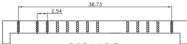
P.C.B LAYOUT
