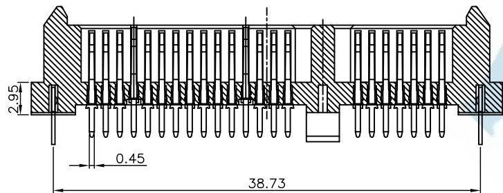
SECT A-A
